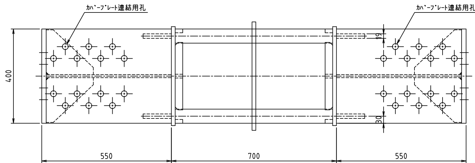
空洞金具詳細図
