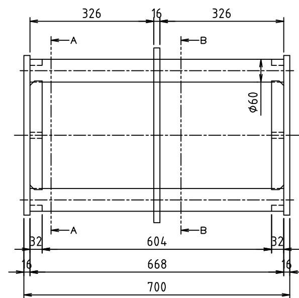
空洞金具詳細図
