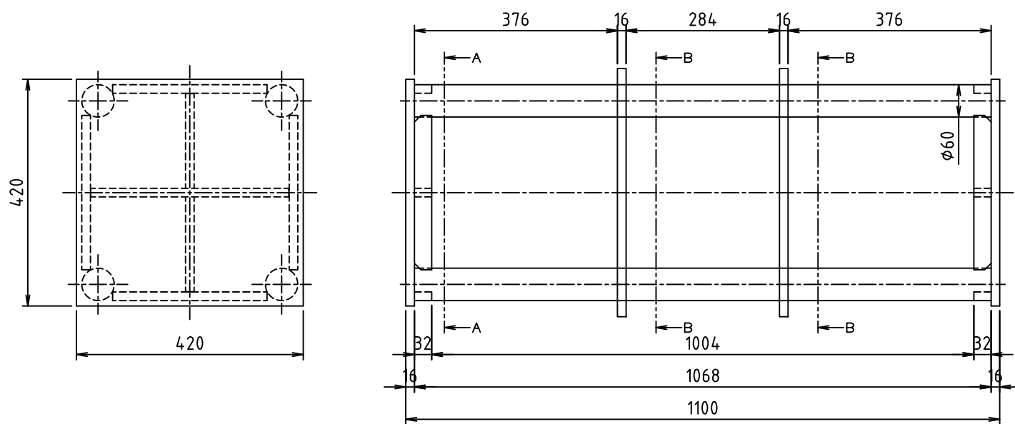
空洞金具詳細図
