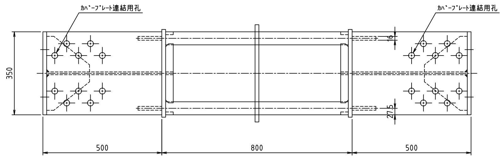
空洞金具詳細図
