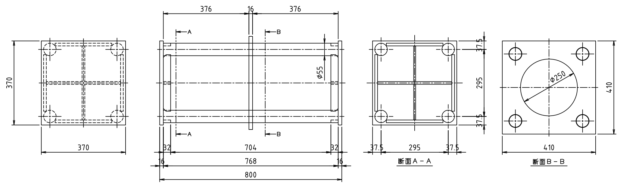
空洞金具詳細図
