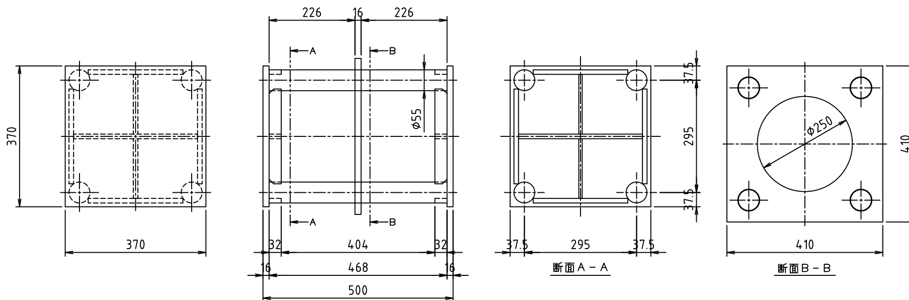
空洞金具詳細図
