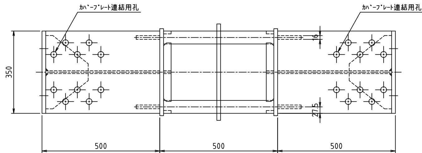
空洞金具詳細図
