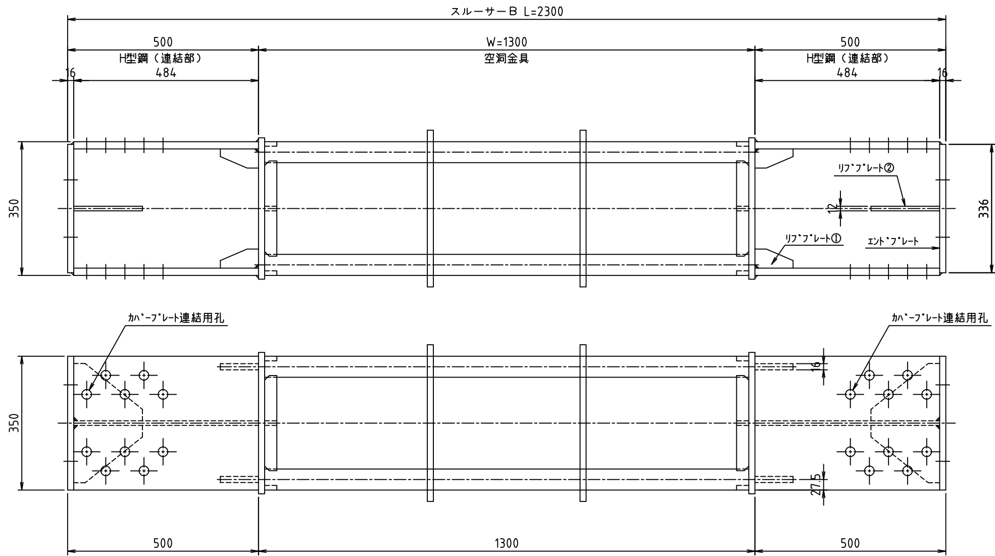
空洞金具詳細図
