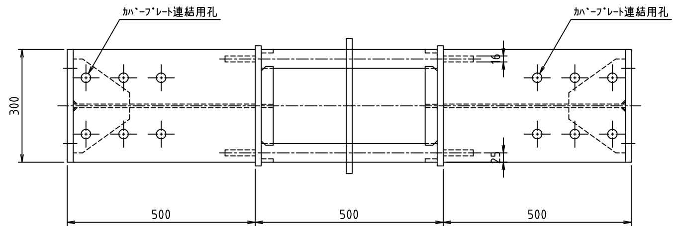
空洞金具詳細図
