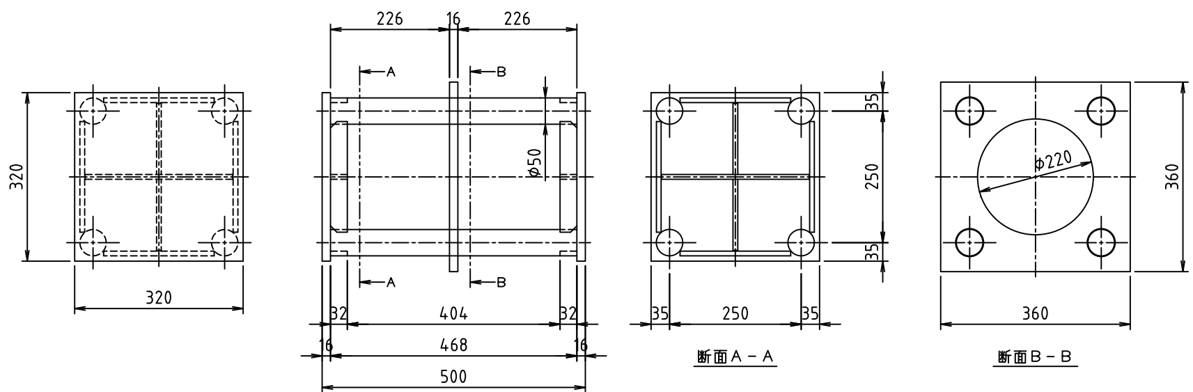
空洞金具詳細図
