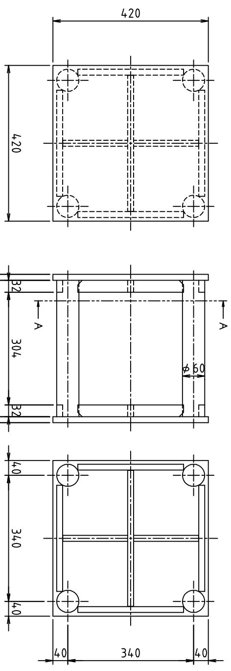
空胴金具詳細図
