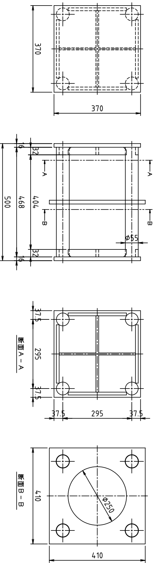
空孔金具詳細図
