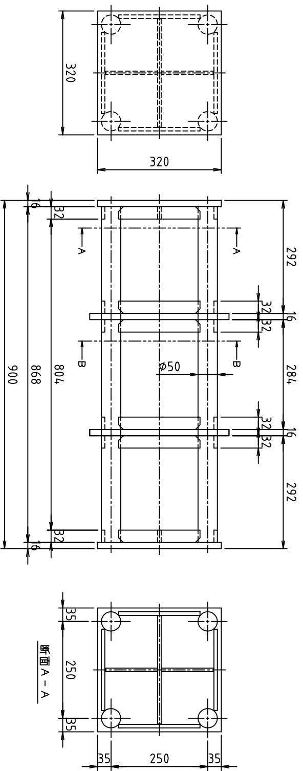
空洞金具詳細図
