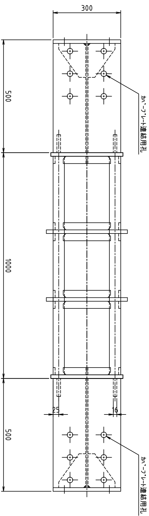
空洞金具詳細図
